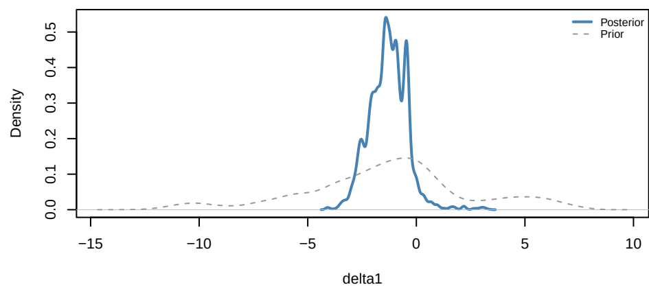
Yasso07 | r
