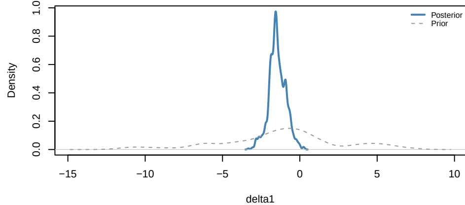
Yasso07 | r
