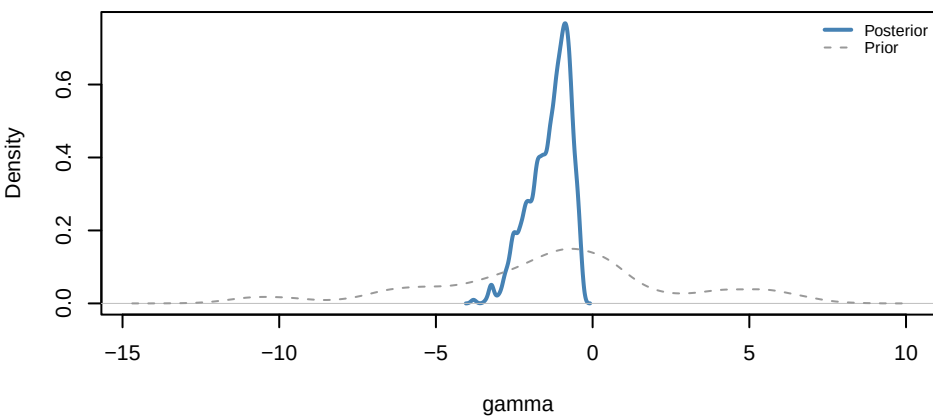
Yasso07 | delta2
