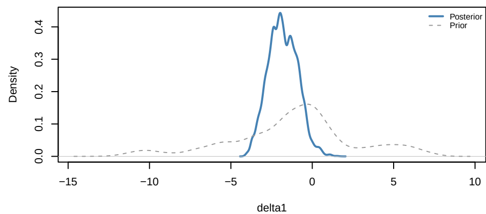
Yasso07 | r
