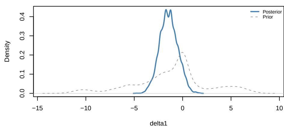
Yasso07 | r
