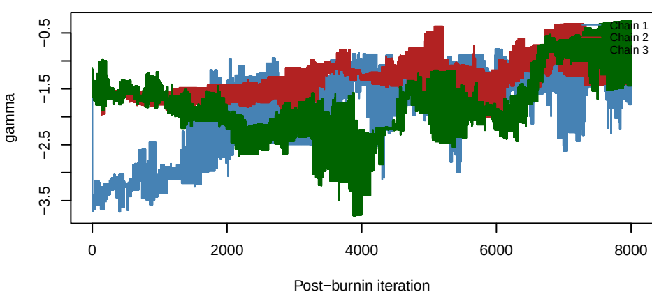
Yasso07 | delta2
