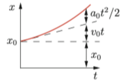
Weg-Zeit-Diagramm
