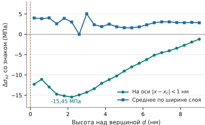
(б) Удерживаемая деформация выступа
