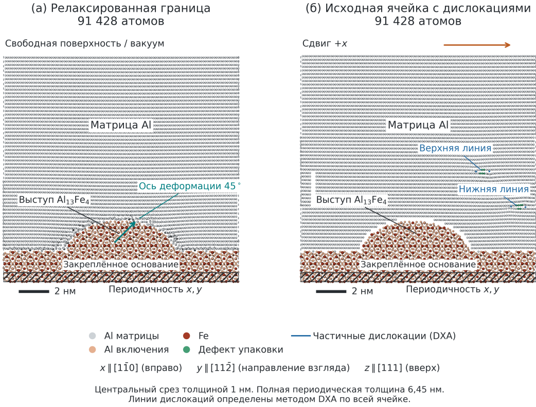
Рис. 1: Атомистическая геометрия границы, визуализированная в OVITO по конфигурациям LAMMPS. Выступ \text{Al}_{13}\text{Fe}_4 протянут вдоль y над плоским опорным слоем. Оси соответствуют направлению скольжения, направлению линии и нормали к границе. Нагружаемая конфигурация содержит пару краевых дислокаций противоположного знака. Верхние слои передают сдвиговую нагрузку, нижний слой закреплён.
