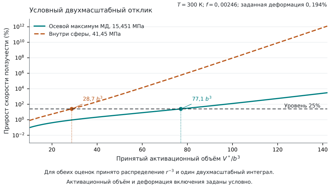
Рис. 4: Условная оценка термически активированного скольжения при 300 К и f = 0,00246 . Амплитуда сдвига, необходимая для прироста скорости на 25%, существенно зависит от активационного объема. Значения 15,451 и 41,45 МПа служат отдельными иллюстративными входными параметрами из профиля выступа и внутреннего поля сферы. Их перенос в скалярную пространственную модель является дополнительным предположением. Кривая не подогнана к измеренному активационному объёму или рассчитанной скорости ползучести.
