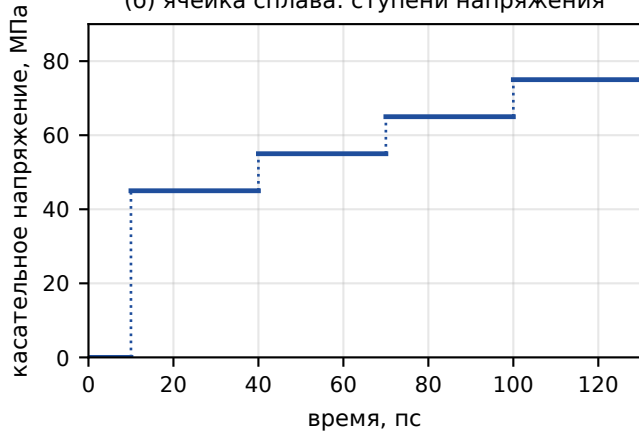
(б) ячейка сплава: ступени напряжения
