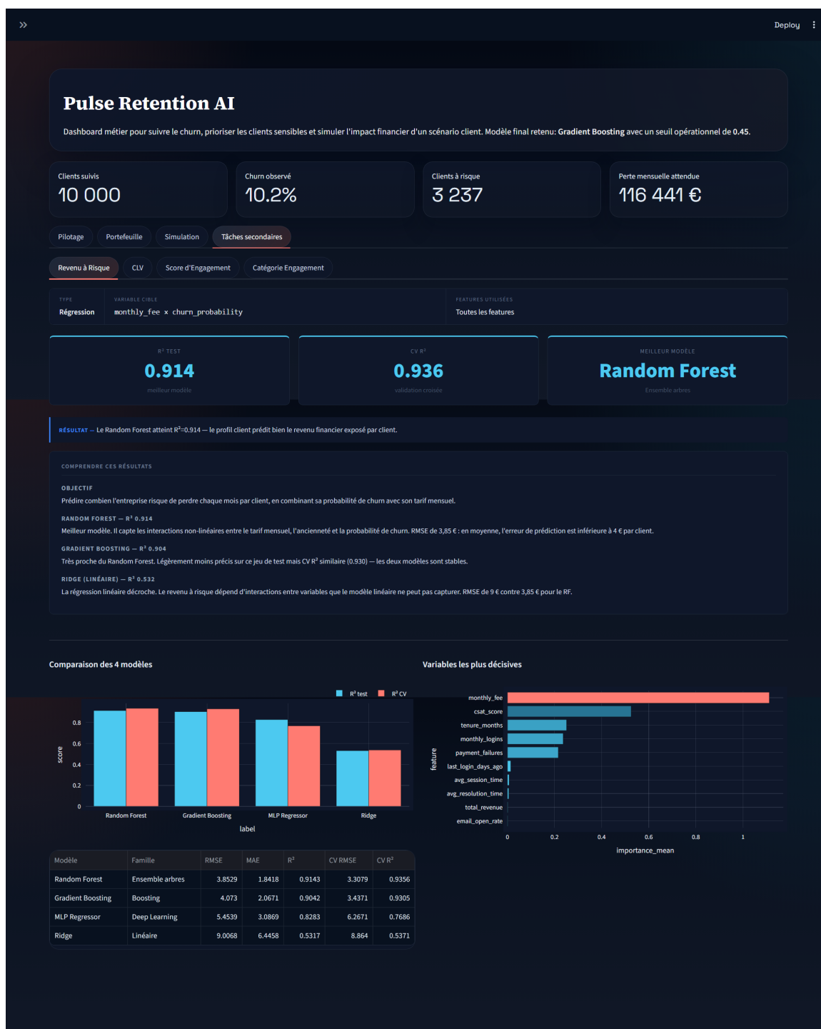
FIGURE 1 – Dashboard — onglet Tâches secondaires : vue complète (sélecteur de tâche, comparaison des 4 modèles, tableau de métriques et feature importance)
