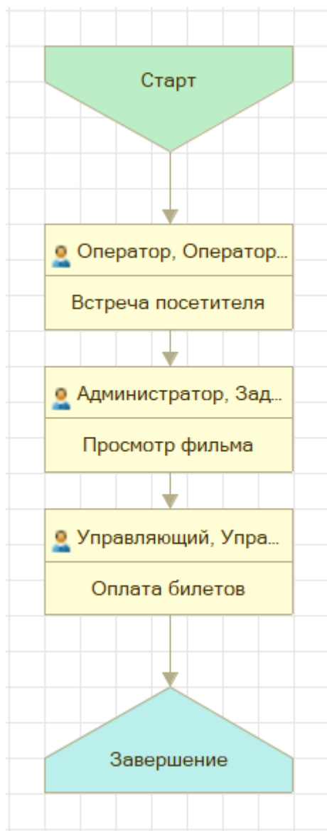
Рисунок 1 – Схема бизнес-процесса
