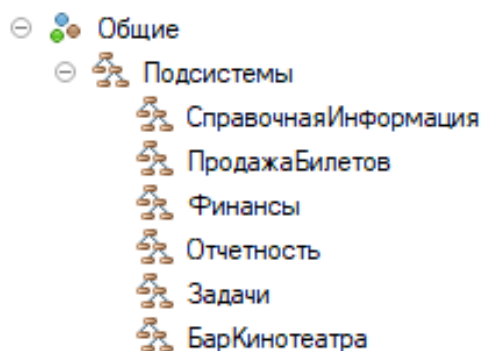
Рисунок 2 – Дерево конфигурации
