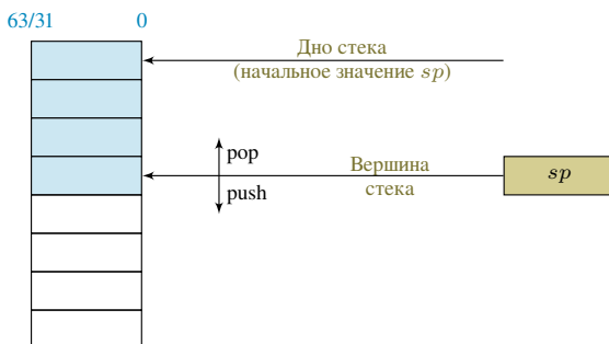
Рис. 3.3. Стек
