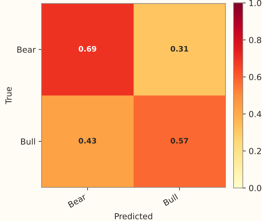
TS2Vec (F1=0.624)
