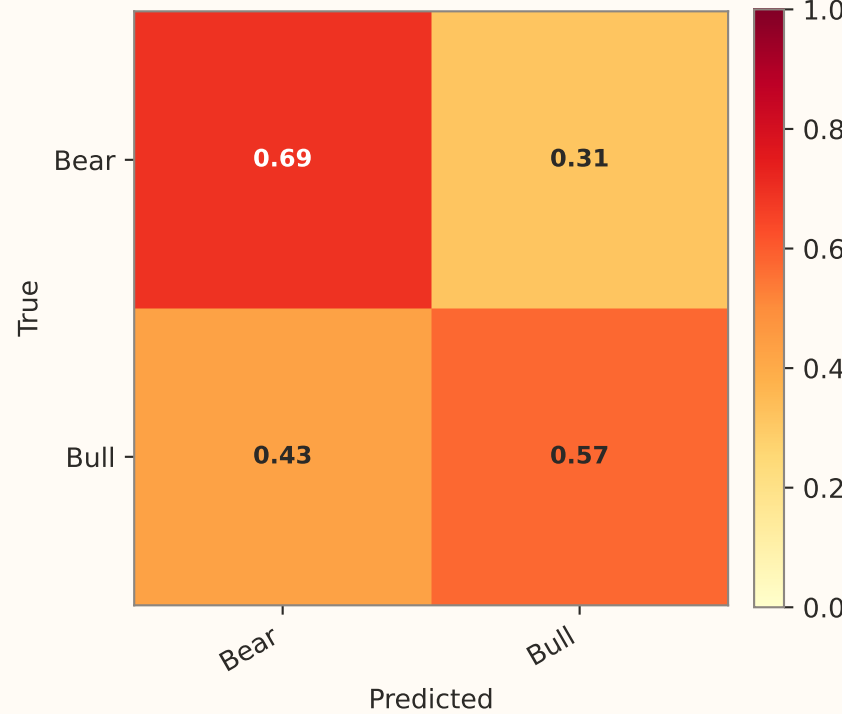
TS2Vec (F1=0.405)
