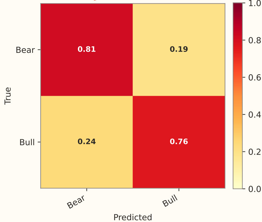
FinJEPA (F1=0.475)
