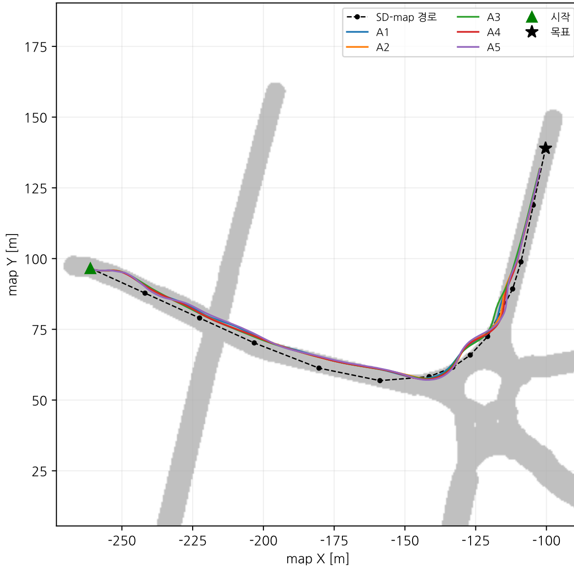
시나리오 4 · 목표 접근 주행 예시
