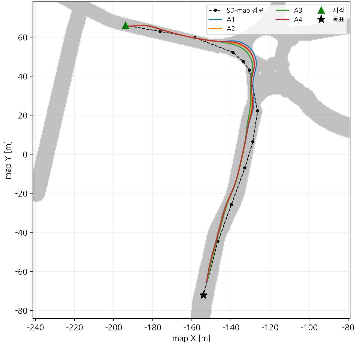
시나리오 6 · 목표 접근 주행 예시
