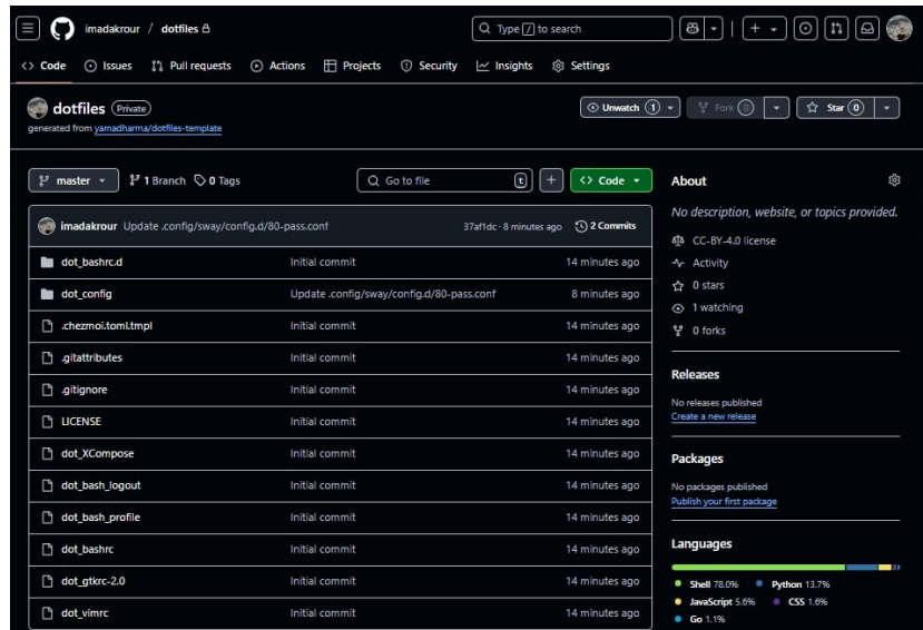
Рис. 4.6: Создание репозитория
