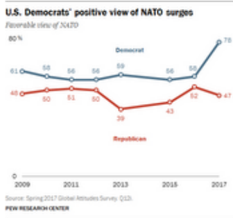
ChartQA
