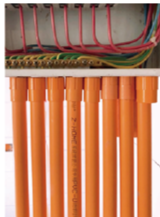
强弱电箱用杯梳连接, 防止线路损坏
