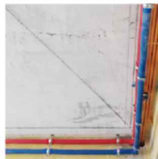
双固定支架加固工艺
