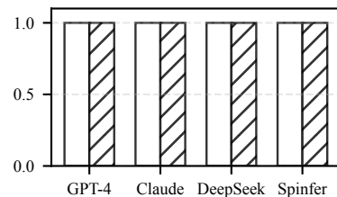
(8) random_ether_addr-84
