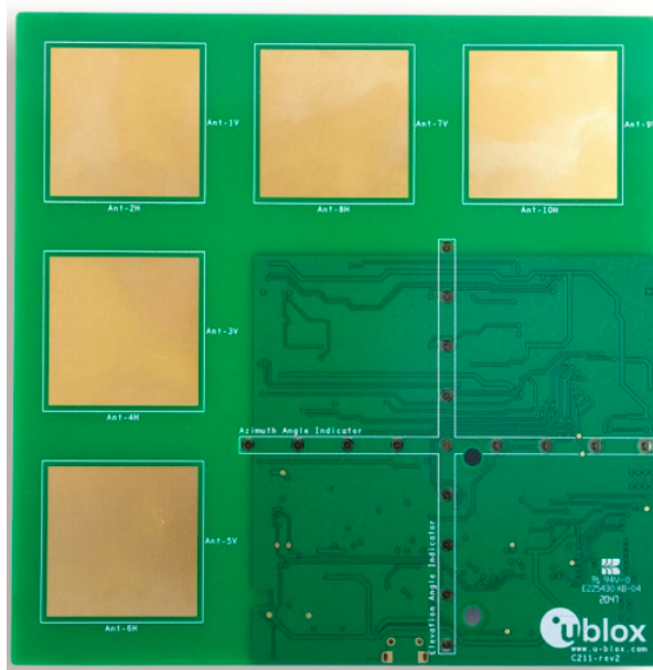
Σχήμα 3.1: XPLR Anchor[10]
