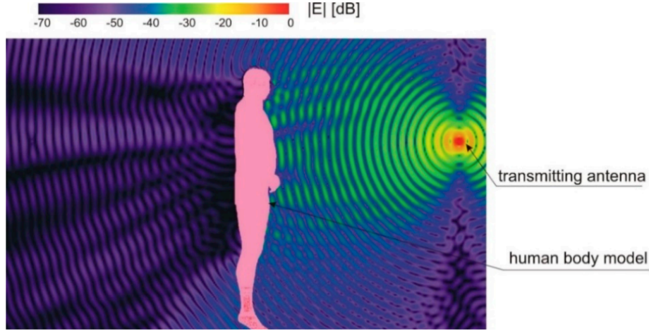
Σχήμα 2.13: Επίδραση Ανθρώπινου Σώματος στην Ισχύ Ραδιοκυμάτων [14]
