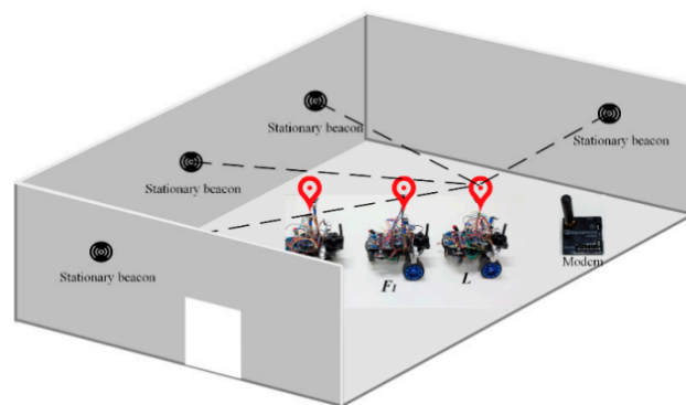
Σχήμα 1.1: Σύστημα Εντοπισμού για Ρομποτικές Εφαρμογές[2]
