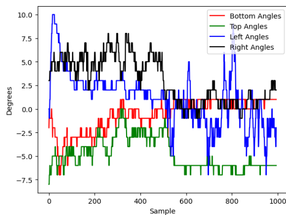
Σχήμα 4.20: Χρονοσειρές γωνιών για το πείραμα 400_170_diag_H_C
