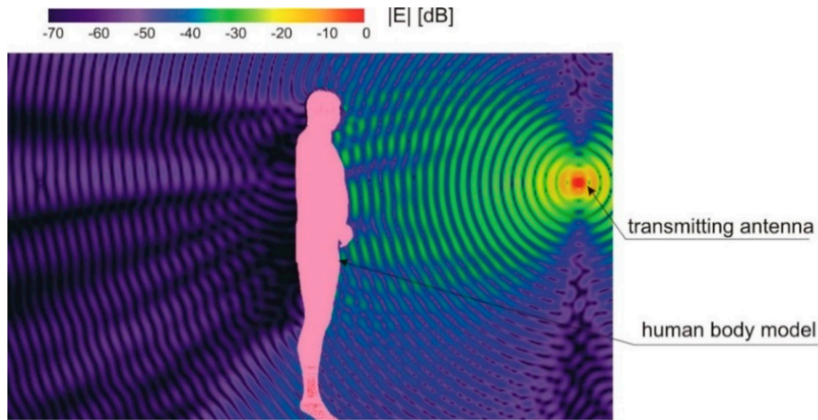
Σχήμα 2.13: Επίδραση Ανθρώπινου Σώματος στην Ισχύ Ραδιοκυμάτων 2.4GHz [15]
