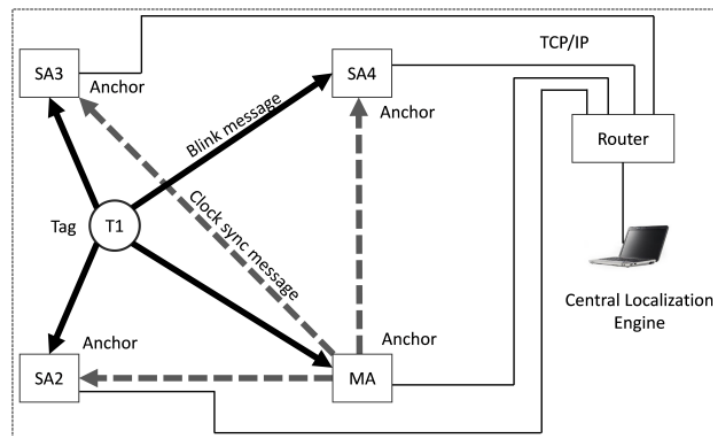
Σχήμα 2.20: Φυσική Αρχιτεκτονική Συστήματος UWB[30]
