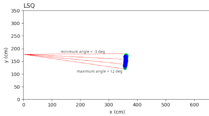
Σχήμα 4.13: Γραφική παράσταση της ταλάντωσης του left anchor
