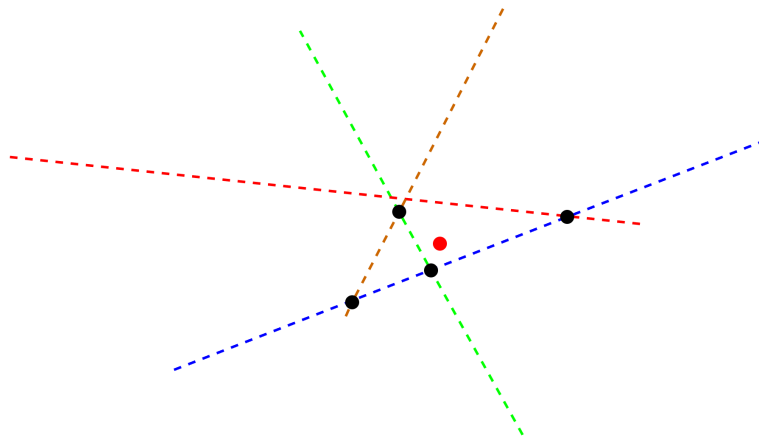
Σχήμα 2.8: Γεωμετρικό Βαρύκεντρο AoA
