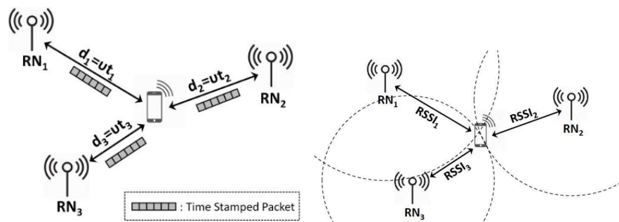
Σχήμα 2.4: Time of Flight και RSSI Trilateration[8]
