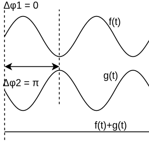
Σχήμα 2.12: Καταστροφική Συμβολή δύο Κυμάτων με Άντίθετες \Delta\phi
