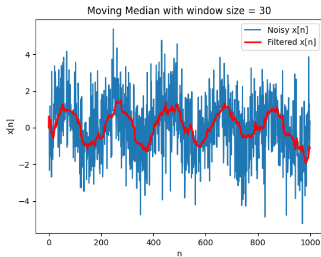
Σχήμα 2.18: Θορυβώδες σήμα φιλτραρισμένο με Moving Median
