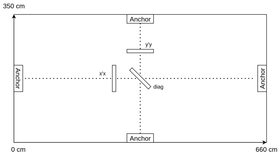
Σχήμα 3.6: Προσανατολισμός του tag ως προς τον άξονα x'x , y'y και διαγώνια
