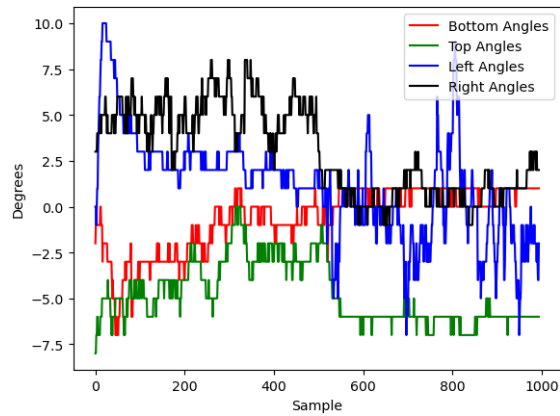
Σχήμα 4.20: Χρονοσειρές γωνιών για τα πείραμα 400_170_diag_H_C
