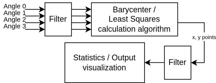
Σχήμα 3.5: Δομή Λογισμικού
