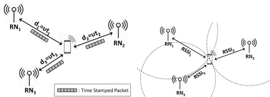
Σχήμα 2.2: Time of Flight και RSSI Trilateration[12]
