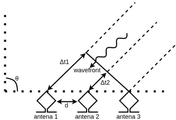
Σχήμα 2.5: Angle of Arrival estimation
