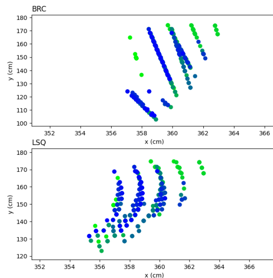
Σχήμα 4.11: Εστιασμένη γραφική παράσταση για το πείραμα 400_170_diag_B
