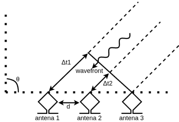
Σχήμα 2.6: Angle of Arrival estimation
