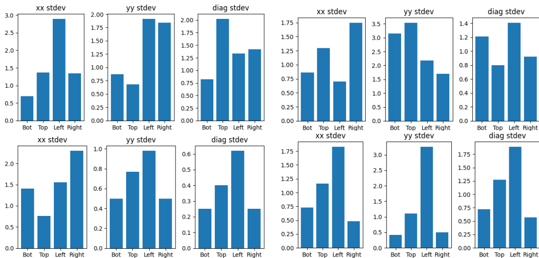
Σχήμα 4.9: Τυπικές αποκλίσεις για τα πειράματα 278_262_A (επάνω αριστερά), 283_168_A (επάνω δεξιά), 400_170_A (κάτω αριστερά) και 504_162_A (κάτω δεξιά) με προσανατολισμούς xx, yy & diag
