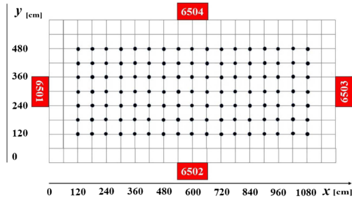
Σχήμα 2.23: Πείραμα στατικών θέσεων σε σύστημα Bluetooth [13]
