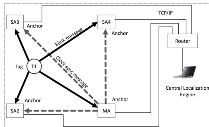
Σχήμα 2.20: Φυσική αρχιτεκτονική συστήματος UWB [31]
