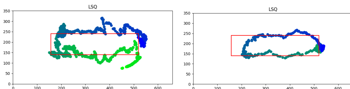
Σχήμα 4.24: Γραφική παράσταση για την κίνηση ορθογώνιου παραλληλόγραμμου, αργή κίνηση (αριστερά) και γρήγορη κίνηση (δεξιά)
