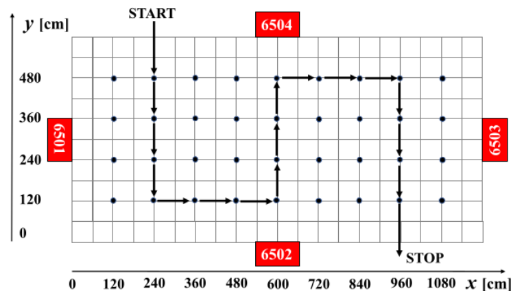
Σχήμα 2.24: Πείραμα κίνησης σε σύστημα Bluetooth [13]
