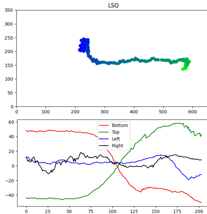
Σχήμα 4.28: Γραφική παράσταση (επάνω) και χρονοσειρές γωνιών (κατώ) για κίνηση δεξιά προς αριστερά με ανθρώπινο εμπόδιο
