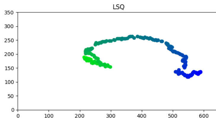
Σχήμα 4.27: Γραφική παράσταση για κίνηση αριστερά προς δεξιά με ανθρώπινο εμπόδιο χωρίς το left anchor
