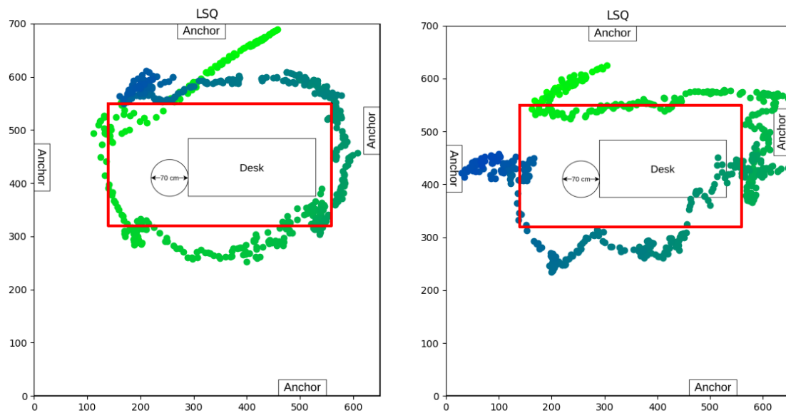
Σχήμα 4.31: Παραλληλόγραμμη κίνηση στο δωμάτιο Β, αριστερόστροφα (αριστερά) και δεξιόστροφα (δεξιά)
