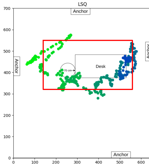
Σχήμα 4.32: Παραλληλόγραμμη κίνηση στο δωμάτιο Β με ανθρώπινο εμπόδιο
