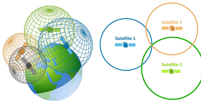
Σχήμα 2.1: GPS Trilateration [2]
