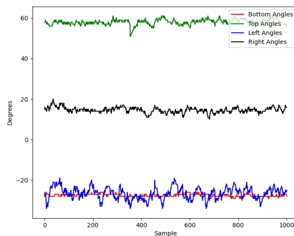
Σχήμα 4.2: Χρονοσειρές γωνιών για το πείραμα 278_262_xx_A
