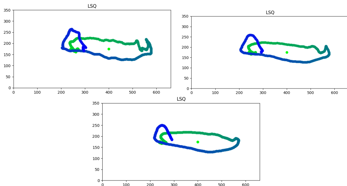
Σχήμα 4.34: Κίνηση παραλληλογράμμου με φιλτράρισμα στις γωνίες για παράθυρο μισού (επάνω αριστερά), ενός (επάνω δεξιά) και δύο δευτερολέπτων (κάτω)
