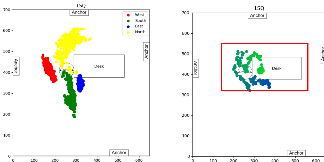
Σχήμα 4.33: Στατικές μετρήσεις (αριστερά) και κυκλική κίνηση (δεξιά) γύρω από την κολώνα
