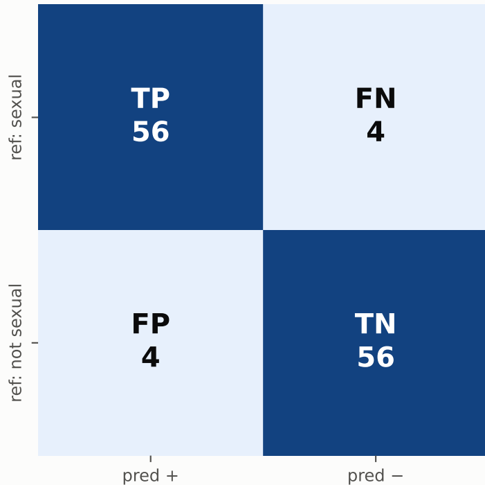
Qwen3.5-9B alone (v3) F1 0.933
