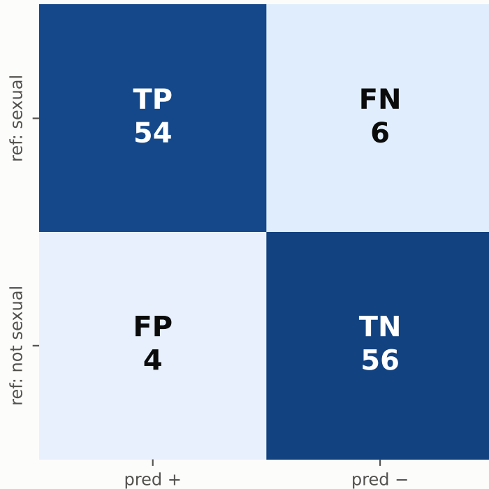
Cascade I_logreg → Qwen v3 (95 %) F1 0.915 · 73 % sent
