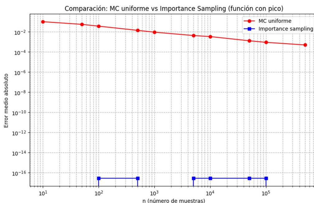
Figura 4. Comparación log-log de MC uniforme e importance sampling para una función con pico. Cuando \rho \propto f , el error del IS es prácticamente nulo.
