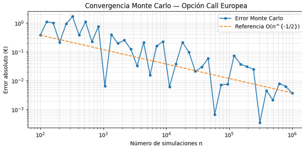
Figura 11. Convergencia Monte Carlo en la valoración de la opción call europea: error absoluto frente al número de simulaciones, comparado con la referencia teórica \mathcal{O}(n^{-1/2}) .
