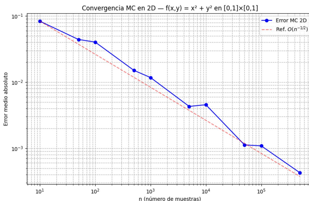
Figura 7. Convergencia del método Monte Carlo en 2D para f(x, y) = x^2 + y^2 en [0, 1] \times [0, 1] . La pendiente en log-log se mantiene próxima a \mathcal{O}(n^{-1/2}) .
