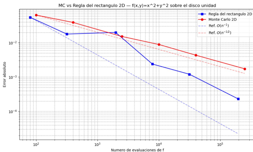
Figura 9. Comparación del error en función del número de evaluaciones para Monte Carlo y regla del rectángulo 2D sobre el disco unidad.
