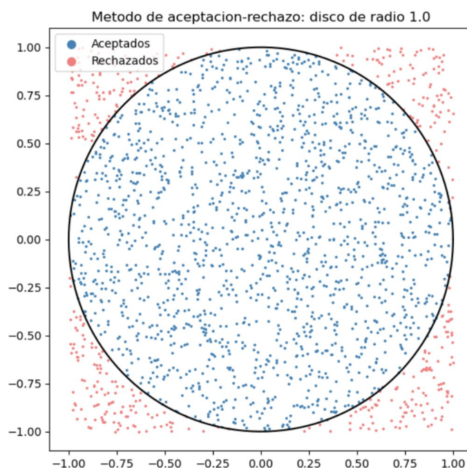
Figura 8. Método de aceptación–rechazo sobre el disco de radio 1: puntos aceptados (azul) y rechazados (rojo).
