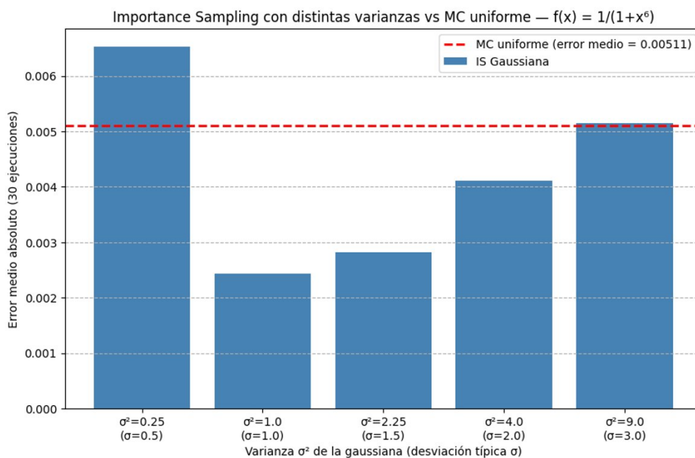
Figura 5. Error medio del importance sampling para distintas varianzas de la gaussiana propuesta, comparado con la línea de referencia del MC uniforme.
