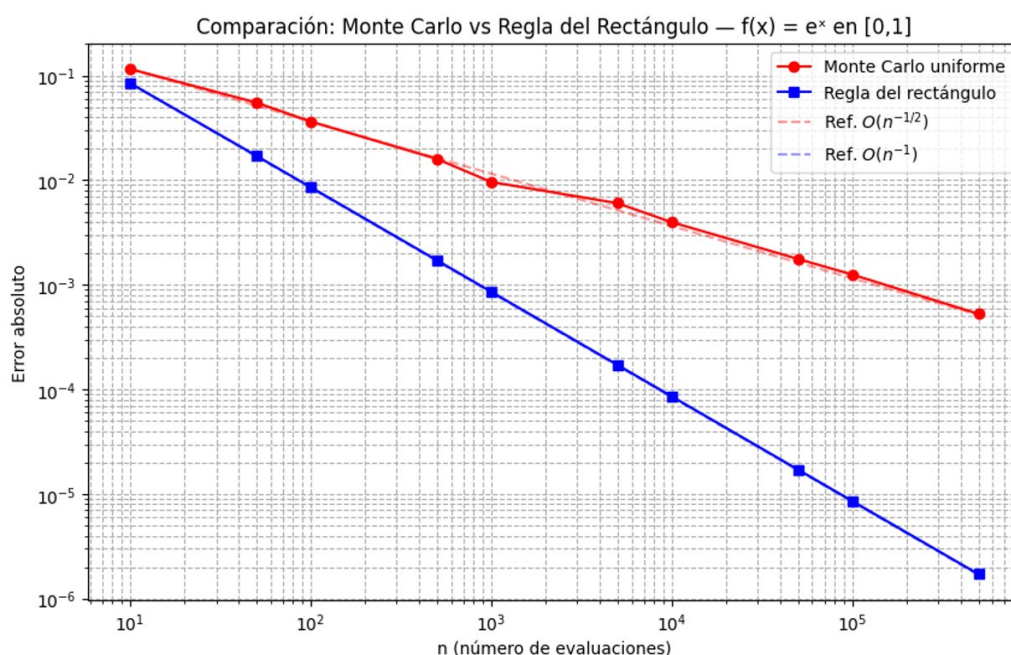
Figura 6. Comparación log-log de Monte Carlo uniforme y regla del rectángulo para f(x) = e^x , junto con las referencias teóricas \mathcal{O}(n^{-1/2}) y \mathcal{O}(n^{-1}) .
