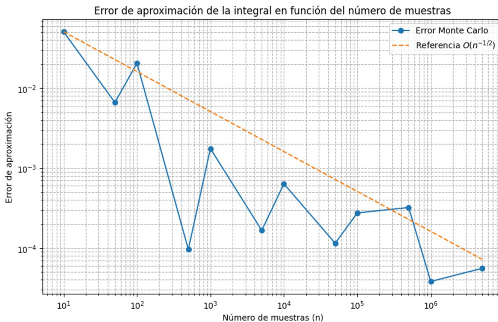
Figura 1. Error de aproximación de la integral en función del número de muestras n (escala log-log). La línea discontinua representa la referencia teórica O(n^{-1/2}) .
