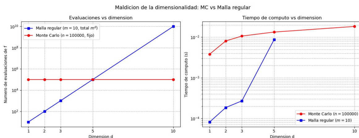
Figura 10. Maldición de la dimensionalidad: evolución del número de evaluaciones (izquierda) y del tiempo de cómputo (derecha) frente a la dimensión, para Monte Carlo y malla regular.
