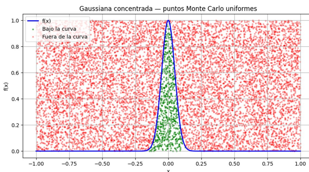
Figura 2. Gaussiana concentrada: los puntos Monte Carlo uniformes (en rojo) caen mayoritariamente fuera de la región donde se concentra el área (en verde).
