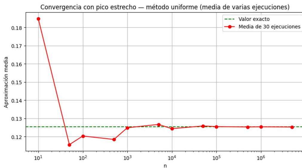
Figura 3. Convergencia del método Monte Carlo uniforme para una gaussiana concentrada: media de 30 ejecuciones frente al valor exacto.
