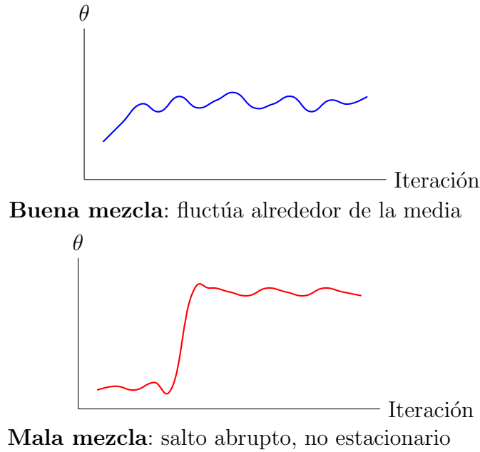
Figura 4: Comparación de trace plots: buena vs. mala convergencia
