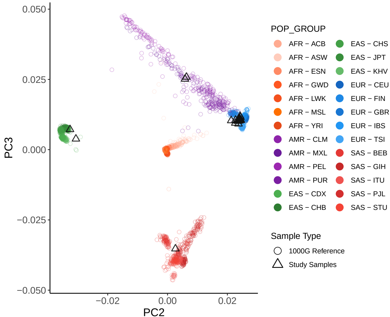
PCA Plot: PC2 vs PC3
