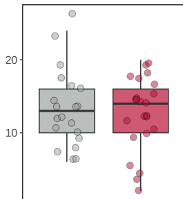
BND
