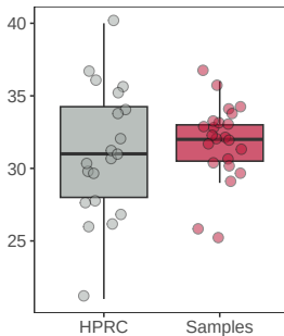
INV
