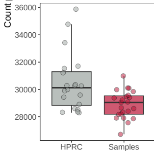
INS
