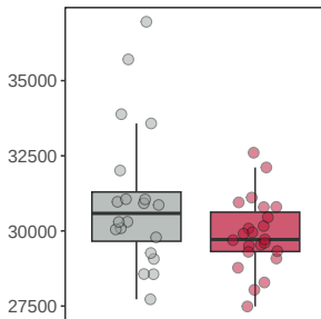
DEL
