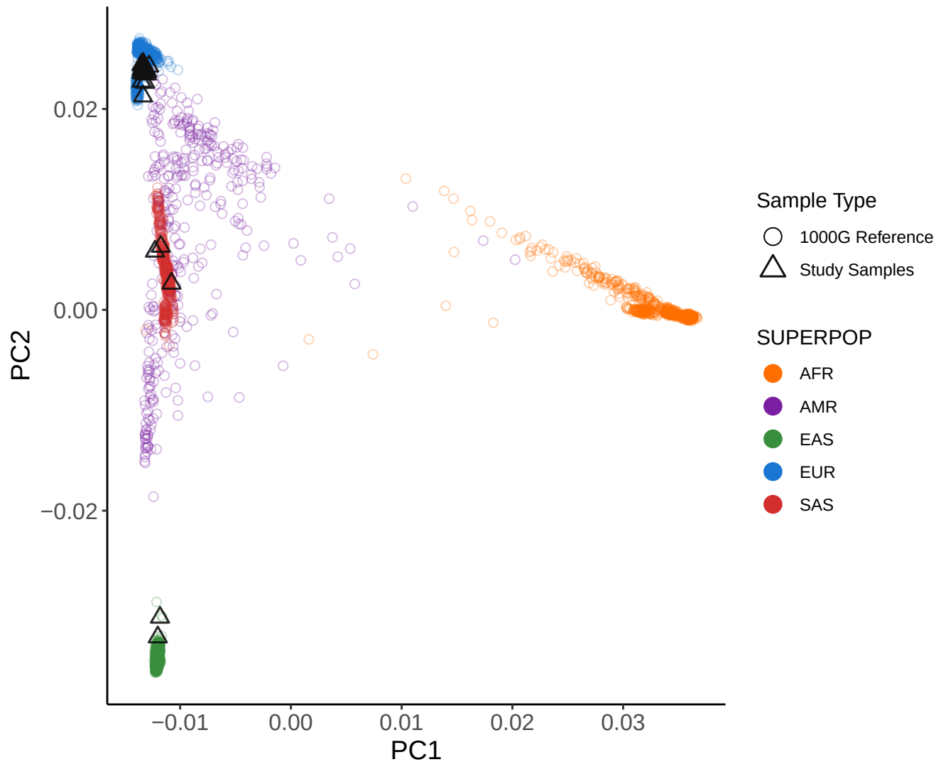
PCA Plot: PC1 vs PC2
