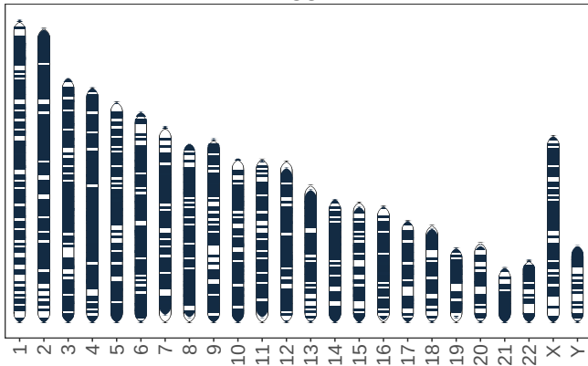
Flagger
