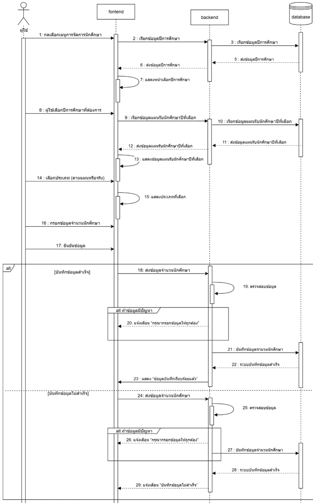
รูปที่ 3. แผนผังการทำงานแบบลำดับปฏิสัมพันธ์
