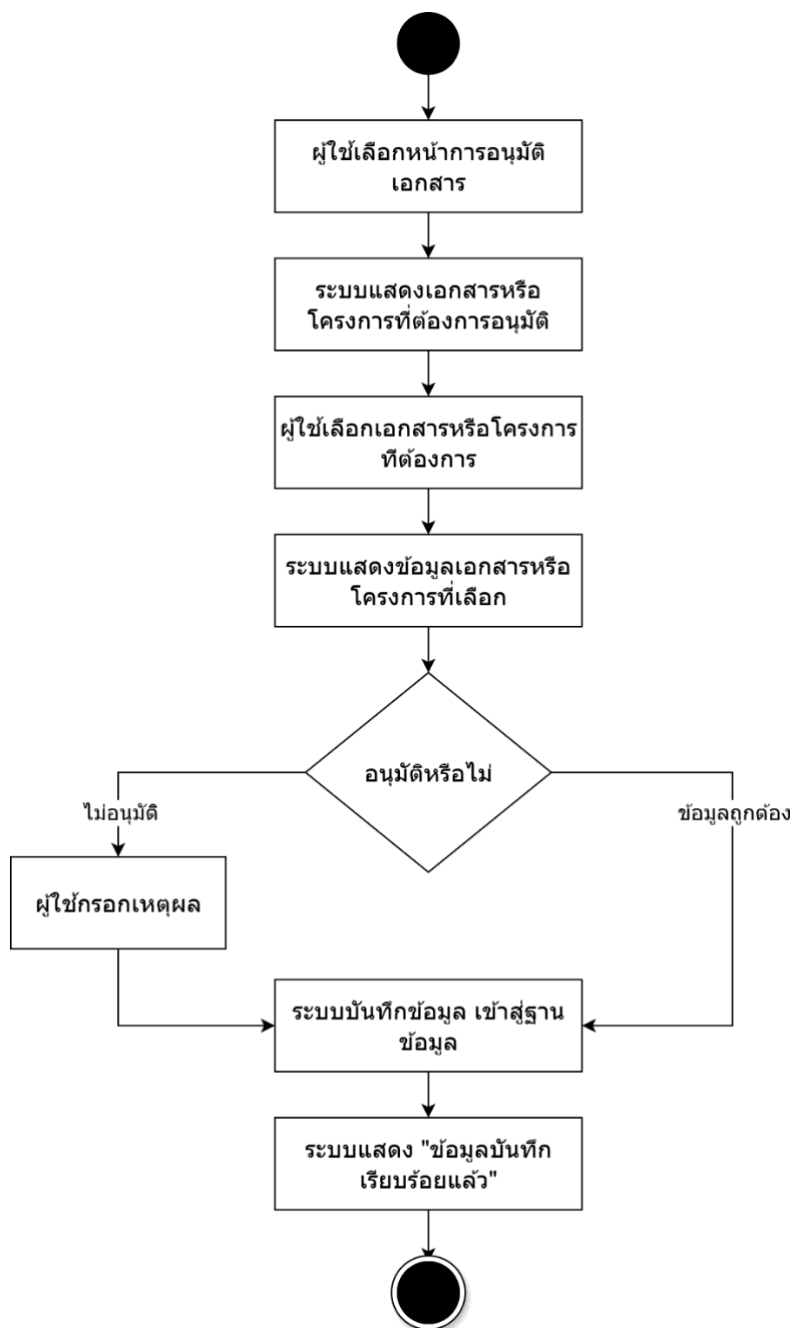
รูปที่ 3. แผนภาพกิจกรรมอนุมัติเอกสารและโครงการ
