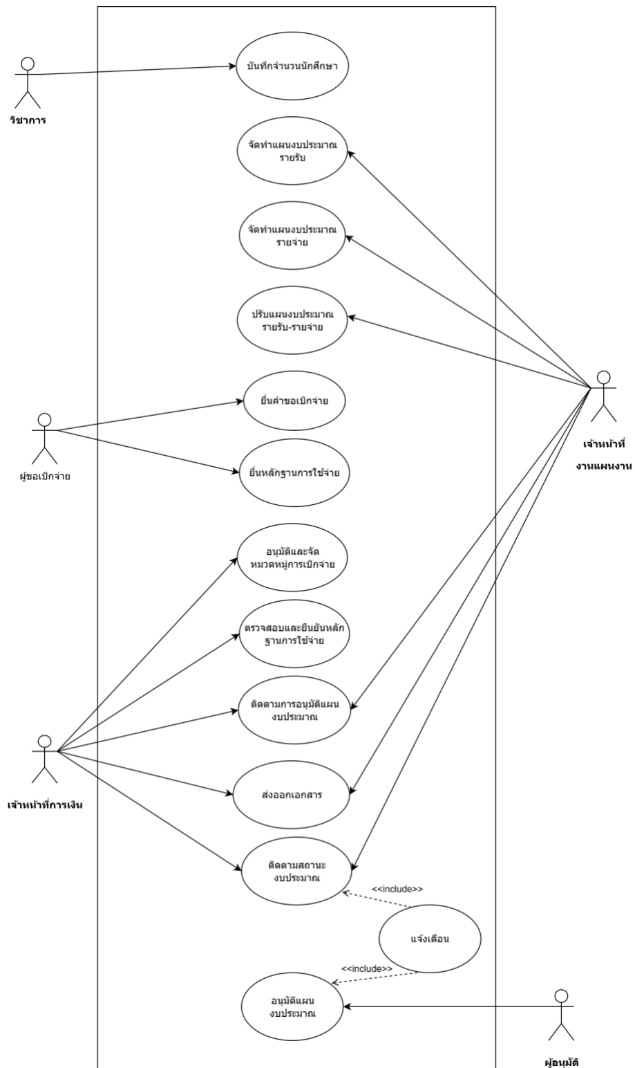
รูปที่ 3.1 แผนภาพยูสเคสของระบบสนับสนุนการจัดทำงบประมาณ
