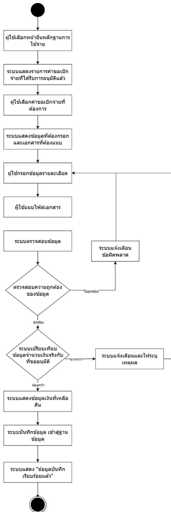
รูปที่ 3. แผนภาพกิจกรรมยื่นหลักฐานการใช้จ่าย
