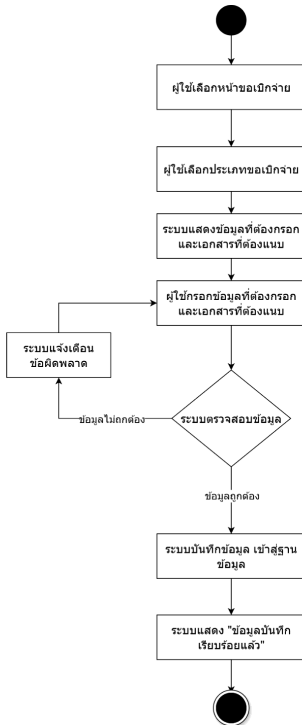
รูปที่ 3. แผนภาพกิจกรรมขอเบิกจ่าย
