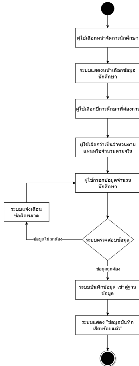
รูปที่ 3. แผนภาพกิจกรรมบันทึกจำนวนนักศึกษา
