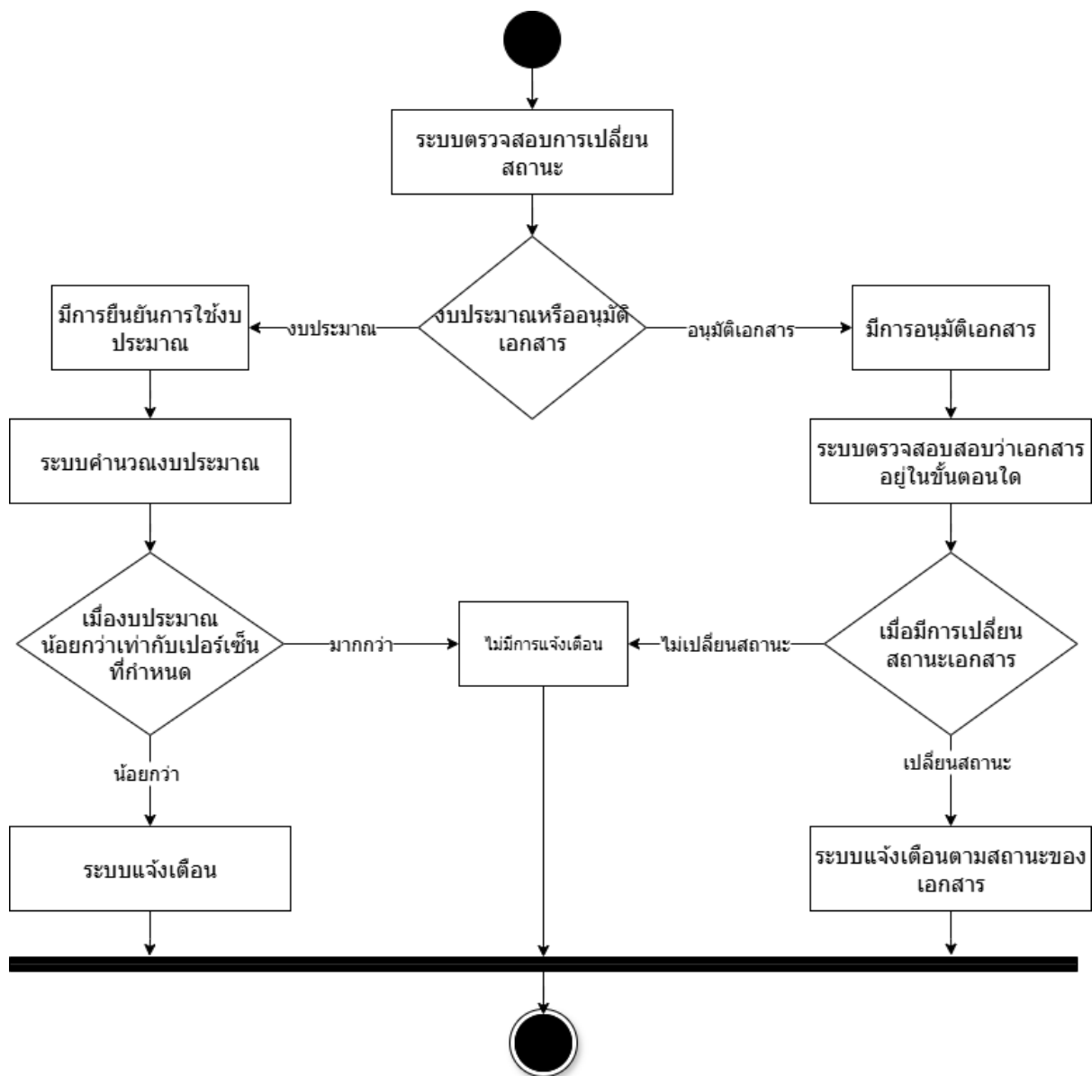
รูปที่ 3. แผนภาพกิจกรรมแจ้งเตือน
