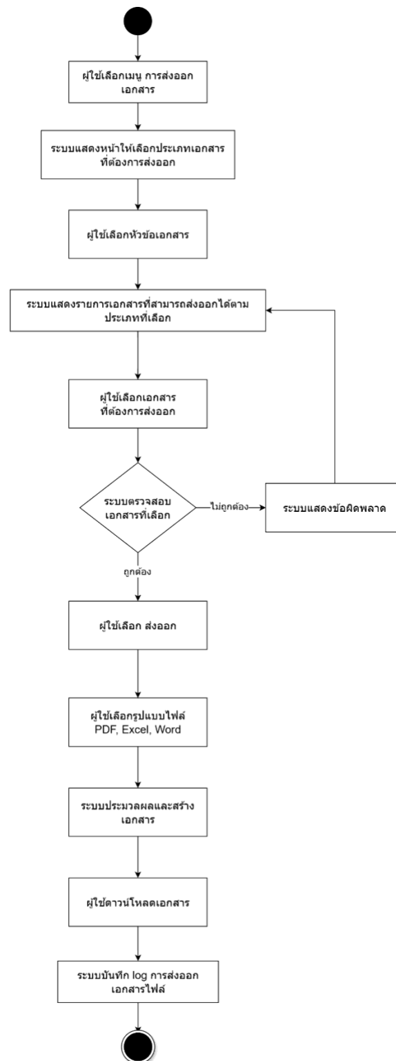
รูปที่ 3. แผนภาพกิจกรรมส่งออกเอกสาร
