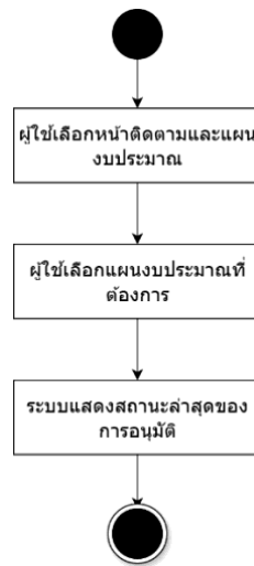
รูปที่ 3. แผนภาพกิจกรรมติดตามการอนุมัติแผนงบประมาณ
