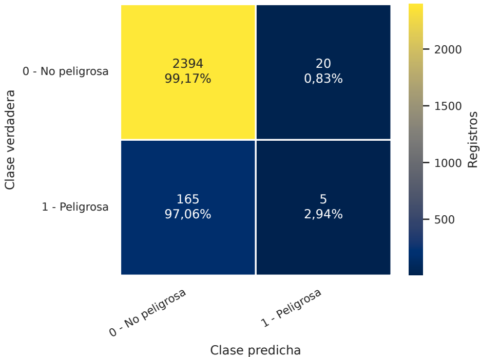
Matriz de confusión: Árbol de decisión base
