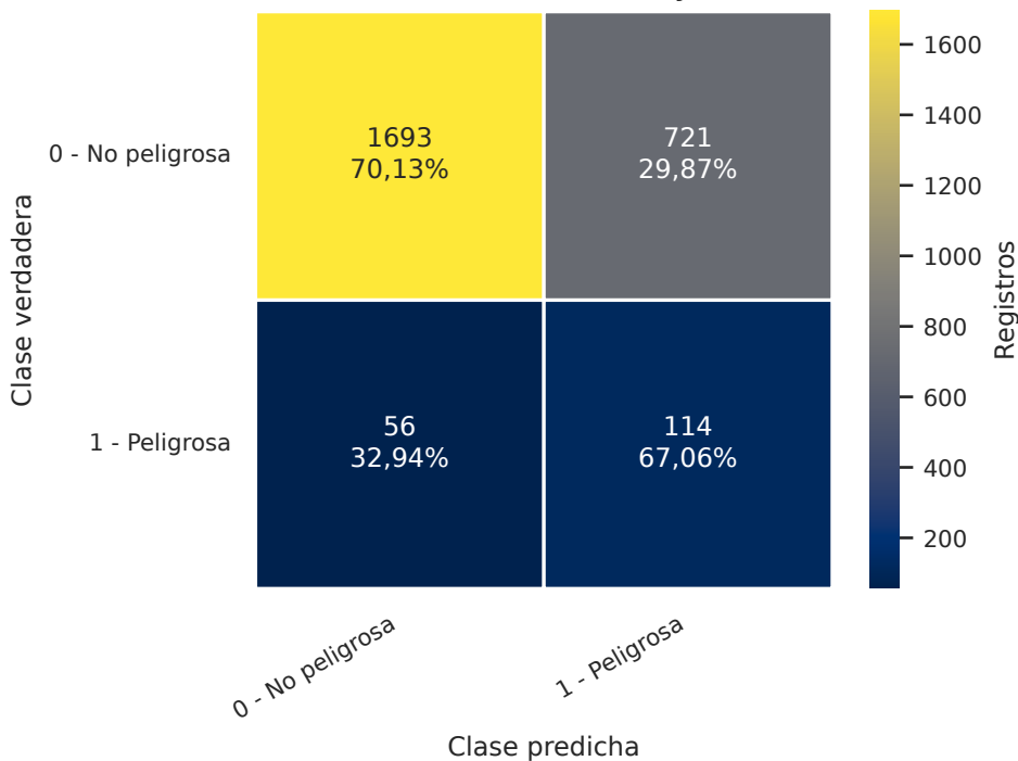
Matriz de confusión: Naive Bayes + SMOTE
