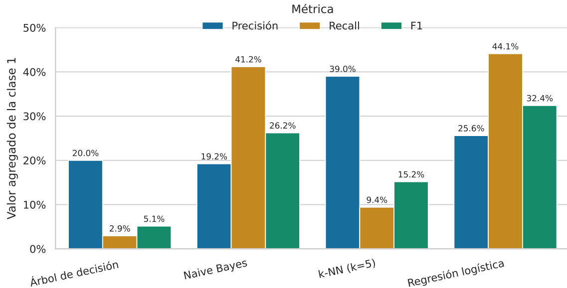
Figura 10: Comparación de la precisión, el recall y el F1 agregados de la clase 1 para los cuatro modelos base.
