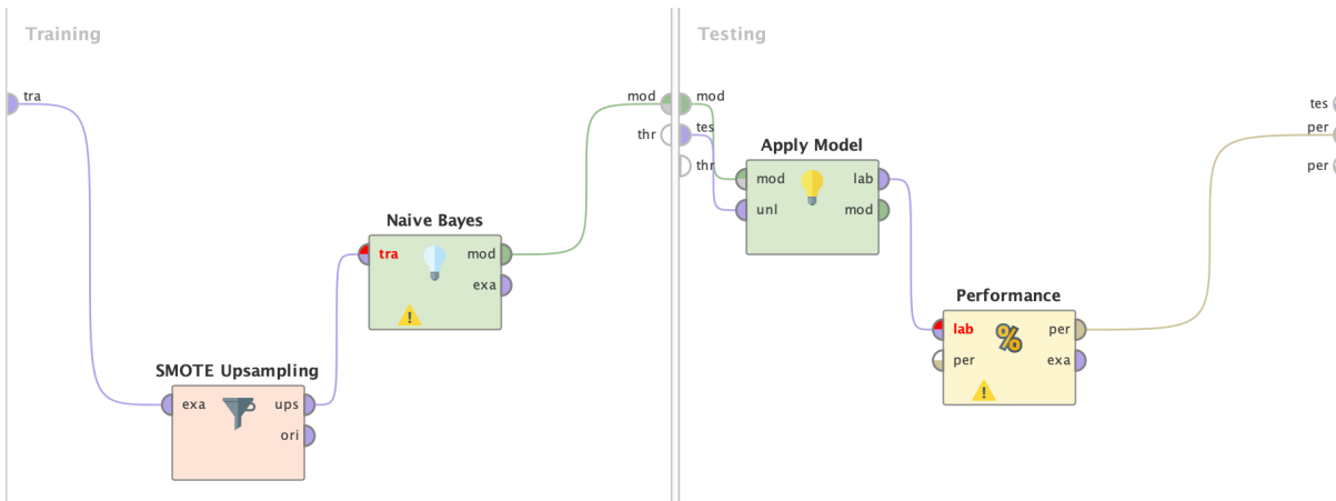
Figura 13: Flujo de Naive Bayes con SMOTE aplicado en Training , seguido de Apply Model y Performance .
