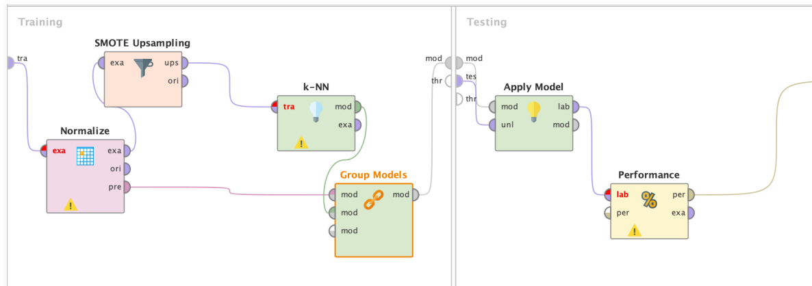
Figura 11: Flujo de k-NN con k = 5 , conservando Normalize antes de SMOTE y aplicando el modelo sobre Testing sin sobremuestreo.
