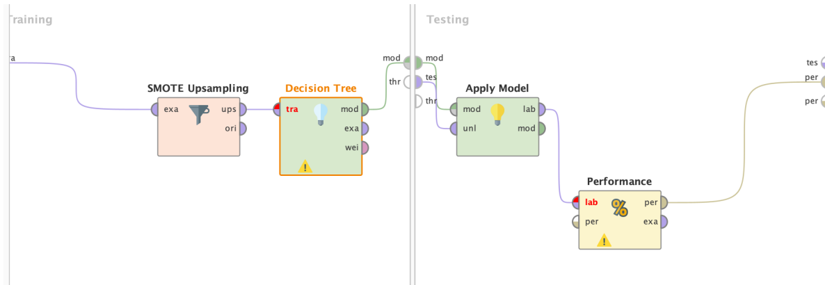
Figura 10: Flujo de árbol de decisión con SMOTE aplicado únicamente en Training , sin incorporar Normalize .
