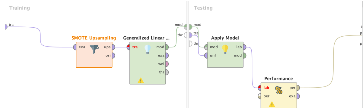
Figura 12: Flujo de regresión logística con SMOTE aplicado únicamente en Training , antes de Generalized Linear Model .
