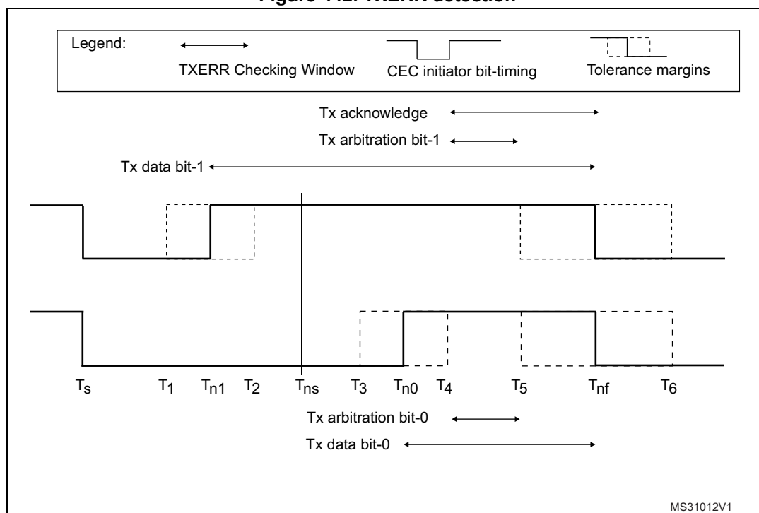
Figure 442. TXERR detection
