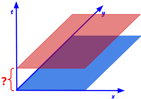
Figura 18 – Qual seria a distância mínima entre duas Bolholândias distintas, para que nenhuma bolha de uma Bolholândia colida com bolhas da outra?
