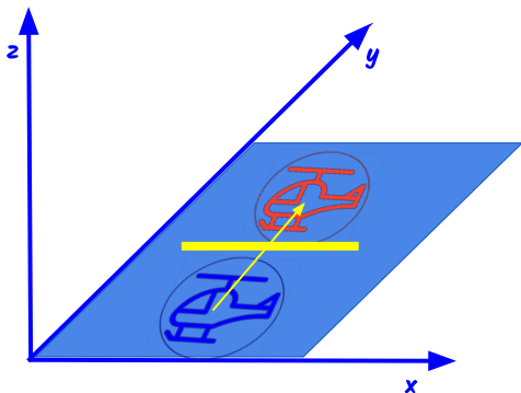
Figura 24 – Nesta visão, o helicóptero bolholandense tenta atravessar um suposto portal unidimensional (1D), representado pela linha amarela, para alcançar outra Bolholândia. No entanto, por ser apenas uma linha, ele o levaria de volta para a mesma realidade de onde partiu.
