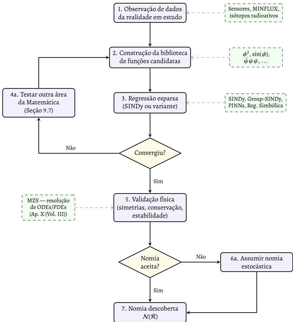
Figura 41 – Fluxograma do processo de descoberta de nomias. O ciclo principal (centro) parte da observação de dados, passa pela construção de bibliotecas funcionais, regressão esparsa e validação física. Se a regressão não convergir com as ferramentas matemáticas disponíveis, explora-se outra área da Matemática (ramo esquerdo). Se a validação falhar repetidamente, pode-se assumir uma nomia estocástica (ramo direito). As ferramentas computacionais (verde, à direita) e o MZS (verde, à esquerda) alimentam as etapas correspondentes.
