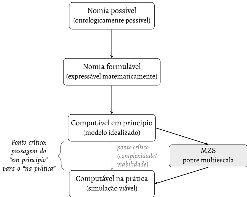
Figura 45 – Fluxo conceitual entre níveis de acessibilidade de uma nomia. A transição entre “computável em princípio” e “computável na prática” representa o ponto crítico onde surgem as principais barreiras analíticas e computacionais. O MZS é indicado como uma ponte metodológica potencial para atuar nessa região.
