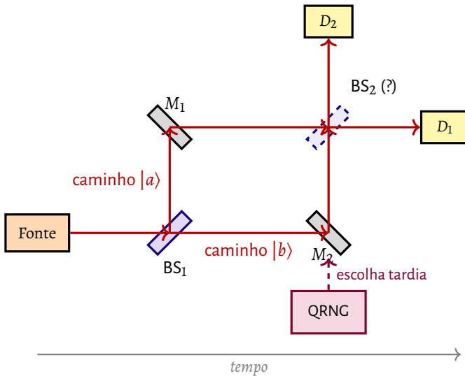
Figura 12 – Esquema do experimento da escolha retardada (versão Mach-Zehnder). Um fóton emitido pela fonte incide no divisor de feixes BS 1 , criando uma superposição coerente dos caminhos |a\rangle (via espelho M 1 ) e |b\rangle (via espelho M 2 ). Decisão crucial: depois que o fóton já passou por BS 1 e está nos braços do interferômetro, um gerador quântico de números aleatórios (QRNG) decide se o segundo divisor BS 2 estará presente ou ausente. Se BS 2 está presente , os caminhos se recombinam e o fóton exibe interferência (comportamento de onda) — detectores D 1 e D 2 registram contagens com probabilidades dependentes da fase relativa entre os braços. Se BS 2 está ausente , cada detector se conecta univocamente a um dos caminhos, revelando trajetória definida (comportamento de partícula). A questão de Wheeler era: como o fóton “sabe” qual comportamento adotar se a decisão foi feita depois que ele já entrou no interferômetro?
